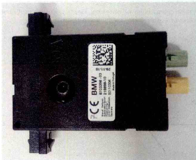
Підсилювач - Вид зверху корпусу (8703398; 8703399)
