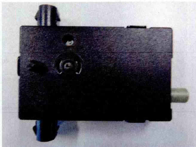
Підсилювач - вид знизу корпусу (8734712; 5A21938)
